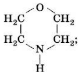
морфолин
